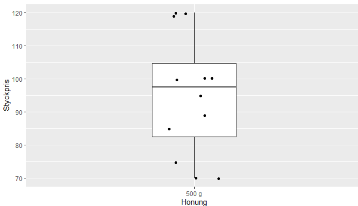
Figur 1. Lådagrammet ger en överblick över prisnoteringarnas spridning för förpackningar med 500 gram honung. Varje prick representerar en prisnotering. De rektangulära lådorna markerar prisintervallet för 50% av de insamlade priserna och den horisontella linjen markerar mittersta värdet (medianen). Priserna inkluderar moms och avser ekologiskt certifierade produkter (EU-ekologisk eller KRAV) som säljs direkt till konsument. Priserna för honung är insamlade under perioden 29 september till 29 oktober 2023, från 9 av Ekologiska Lantbrukarnas 19 distrikt.
