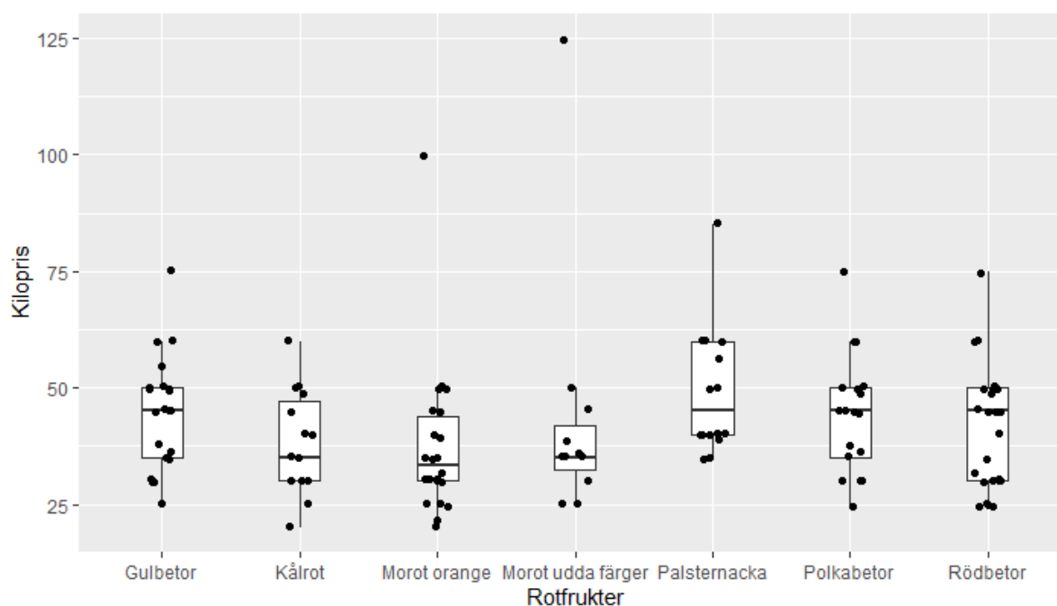
Figur 3. Lådagrammet ger en överblick över prisnoteringarnas spridning uppdelat efter de olika rotfrukterna: morot (orange), morot (udda färger), palsternacka, rödbetor, gulbetor, polkabetor och kålröt. Varje prick representerar en prisnotering. De rektangulära lådorna markerar prisintervallet för 50% av de insamlade priserna och den horisontella linjen markerar mittersta värdet (medianen). Priserna inkluderar moms och avser ekologiskt certifierade produkter (EU-ekologisk eller KRAV) som säljs direkt till konsument. Priserna för grönsaker är insamlade under perioden 29 september till 29 oktober 2023, från 15 av Ekologiska Lantbrukarnas 19 distrikt.
