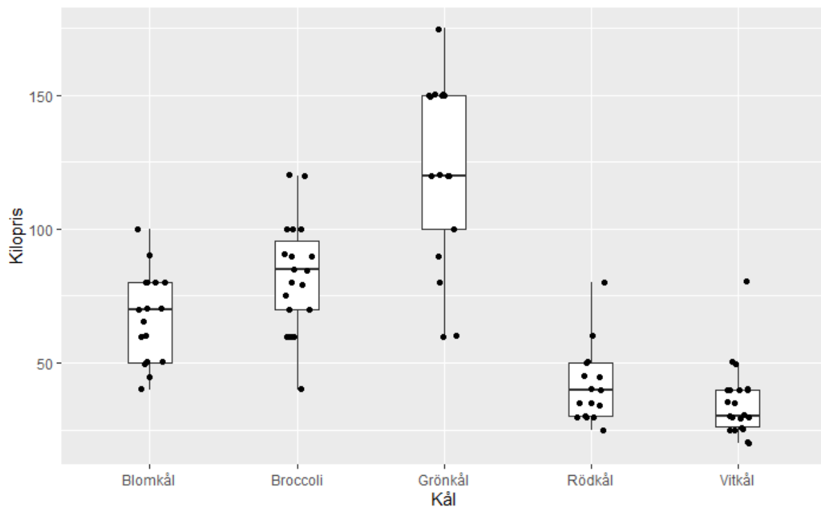
Figur 4. Lådagrammet ger en överblick över prisnoteringarnas spridning uppdelat efter de olika kålsorterna: blomkål, broccoli, grönkål, vitkål och rödkål. Varje prick representerar en prisnotering. De rektangulära lådorna markerar prisintervallet för 50% av de insamlade priserna och den horisontella linjen markerar mittersta värdet (medianen). Priserna inkluderar moms och avser ekologiskt certifierade produkter (EU-ekologisk eller KRAV) som säljs direkt till konsument. Priserna för grönsaker är insamlade under perioden 29 september till 29 oktober 2023, från 15 av Ekologiska Lantbrukarnas 19 distrikt.
