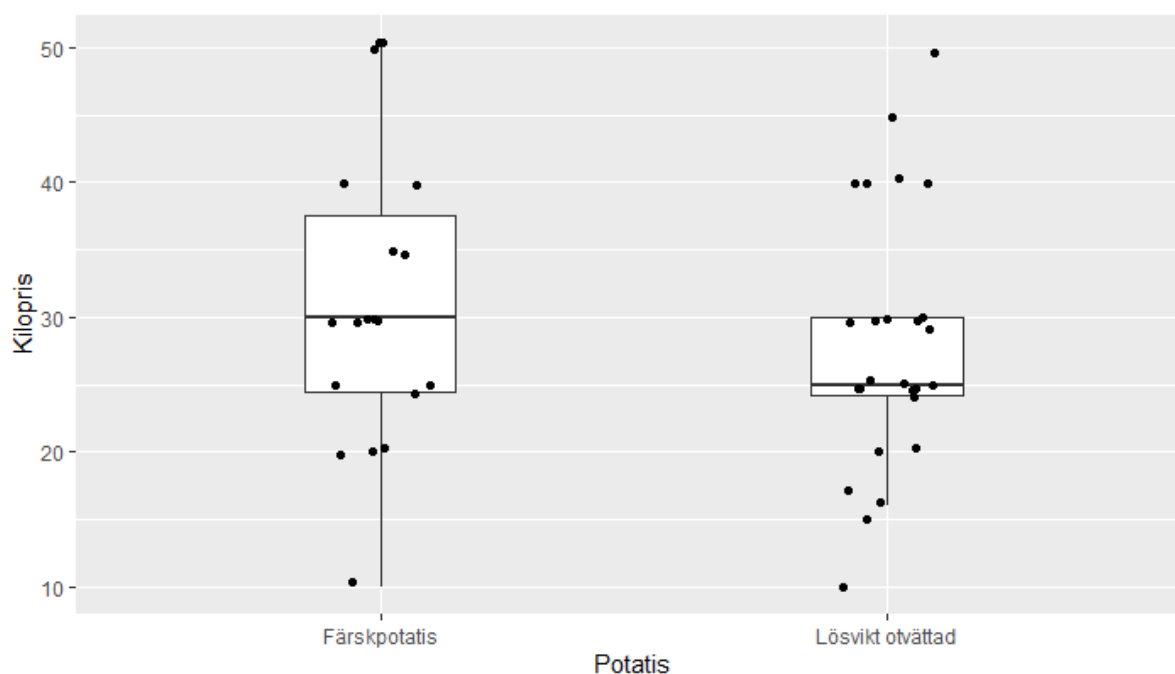
Figur 1. Lådagrammet ger en överblick över prisnoteringarnas spridning uppdelat efter färskpotatis respektive otvättad lösviktspotatis. Varje prick representerar en prisnotering. De rektangulära lådorna markerar prisintervallet för 50% av de insamlade priserna och den horisontella linjen markerar mittersta värdet (medianen). Priserna inkluderar moms och avser ekologiskt certifierade produkter (EU-ekologisk eller KRAV) som säljs direkt till konsument. Priserna för grönsaker är insamlade under perioden 29 september till 29 oktober 2023, från 15 av Ekologiska Lantbrukarnas 19 distrikt.
