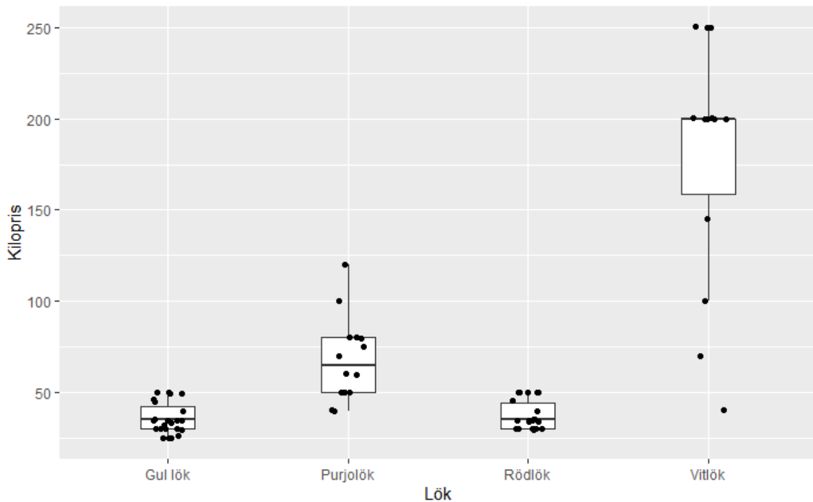
Figur 5. Lådagrammet ger en överblick över prisnoteringarnas spridning uppdelat efter respektive löksort: gul lök, rödlök, vitlök och purjolök. Varje prick representerar en prisnotering. De rektangulära lådorna markerar prisintervallet för 50% av de insamlade priserna och den horisontella linjen markerar mittersta värdet (medianen). Priserna inkluderar moms och avser ekologiskt certifierade produkter (EU-ekologisk eller KRAV) som säljs direkt till konsument. Priserna för grönsaker är insamlade under perioden 29 september till 29 oktober 2023, från 15 av Ekologiska Lantbrukarnas 19 distrikt.
